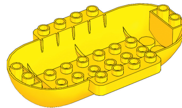
1x 6470277
